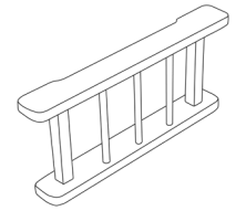
ARMREST W57 D8 H25
